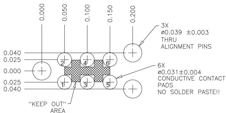
PCB TOP LAYER
