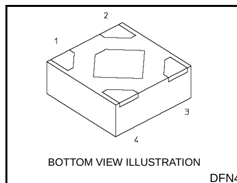
Weight : 1.3 mg ( typ.)
