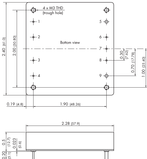
TEP 75 module
