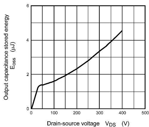
Fig. 8.10 E_{oss} - V_{DS}
