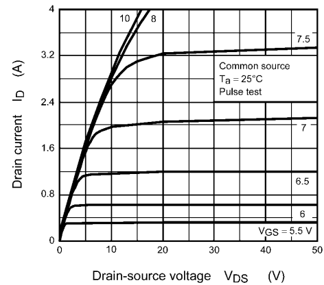
Fig. 8.2 I_D - V_{DS}
