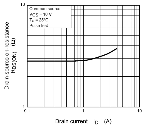
Fig. 8.6 R_{DS(ON)} - I_D
