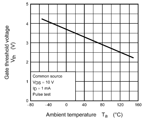
Fig. 8.10 V_{th} - T_a
