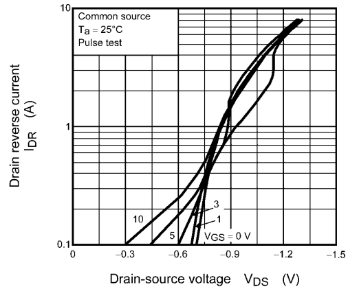
Fig. 8.8 I_{DR} - V_{DS}
