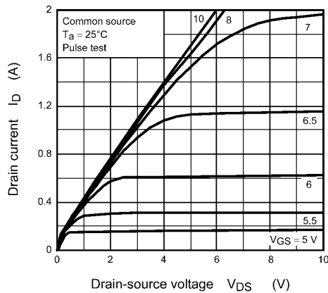
Fig. 8.1 I_D - V_{DS}
