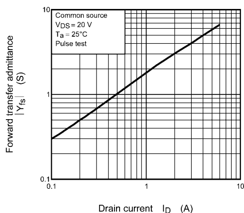
Fig. 8.5 |Y_{fs}| - I_D
