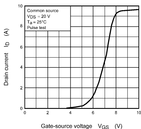
Fig. 8.3 I_D - V_{GS}
