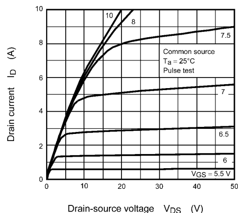
Fig. 8.2 I_D - V_{DS}
