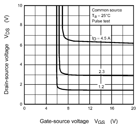
Fig. 8.4 V_{DS} - V_{GS}
