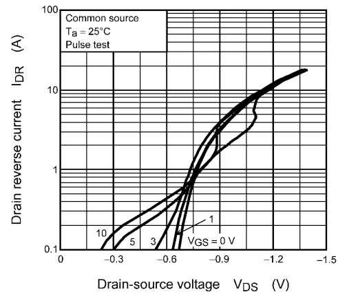
Fig. 8.8 I_{DR} - V_{DS}
