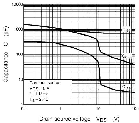
Fig. 8.9 C - V_{DS}
