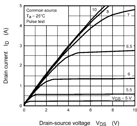
Fig. 8.1 I_D - V_{DS}
