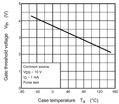
Fig. 8.10 V_{th} - T_a
