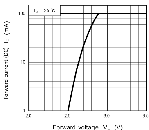
Fig. 8.1 I_F - V_F
