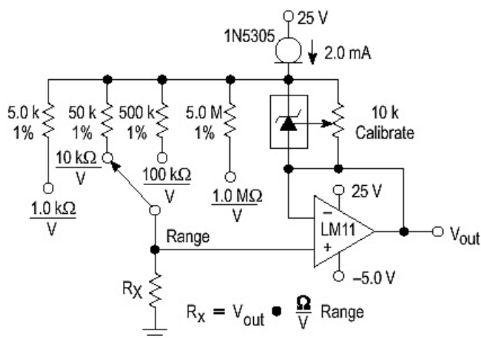
Fig 17.Liner ohmmeter
