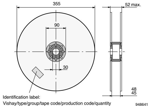
Fig. 7 - Reel Dimensions
