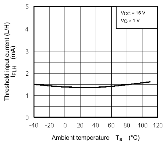
Fig. 12.2.3 I_{FLH} - T_a
