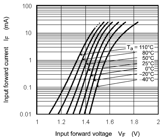
Fig. 12.2.1 I_F - V_F
