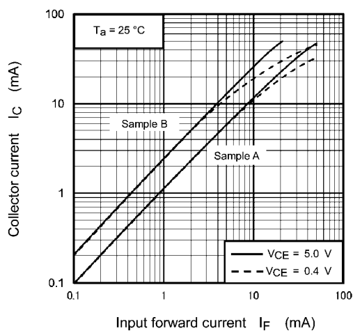
Fig. 11.9 I_C - I_F
