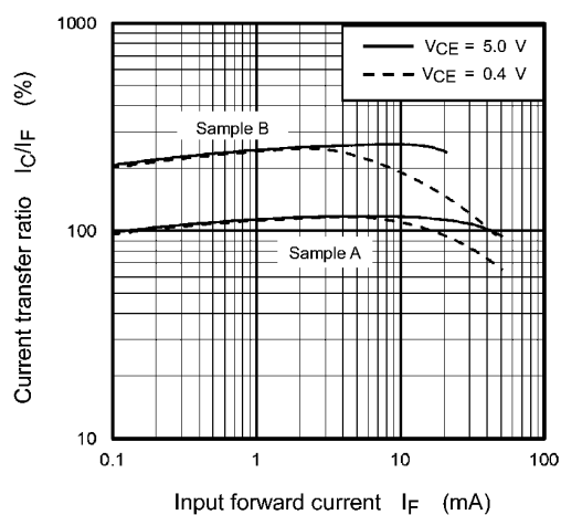
Fig. 11.10 I_C/I_F - I_F
