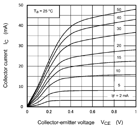
Fig. 11.8 I_C - V_{CE}
