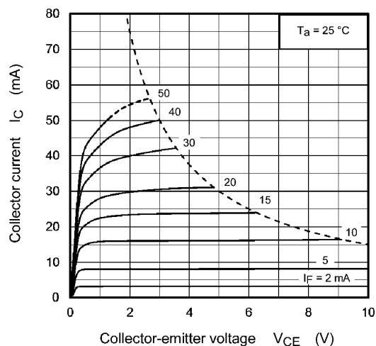
Fig. 11.7 I_C - V_{CE}
