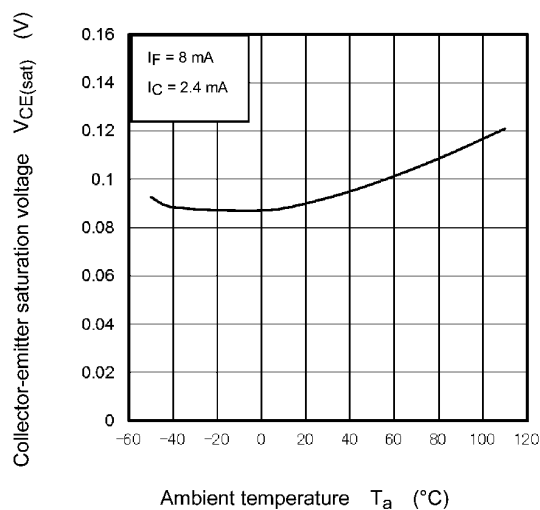
Fig. 11.12 V_{CE(sat)} - T_a
