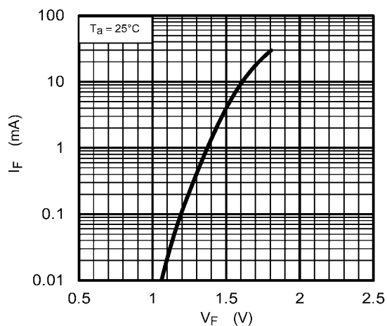
Fig. 13.1.3 I_F - V_F
