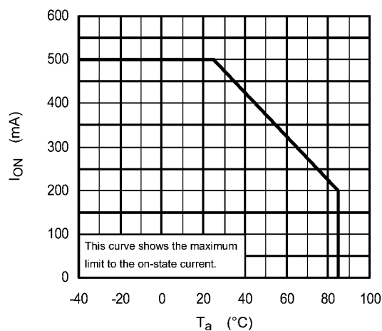
Fig. 13.1.2 I_{ON} - T_a
