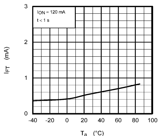
Fig. 14.1.6 I_{FT} - T_a
