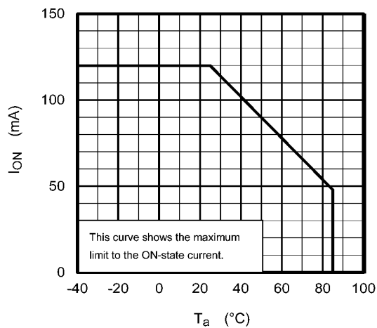
Fig. 14.1.2 I_{ON} - T_a
