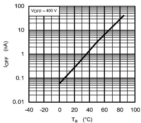
Fig. 14.1.9 I_{OFF} - T_a
