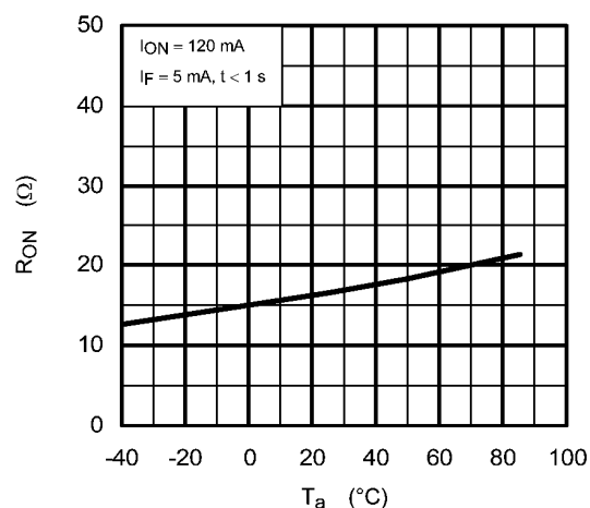
Fig. 14.1.5 R_{ON} - T_a
