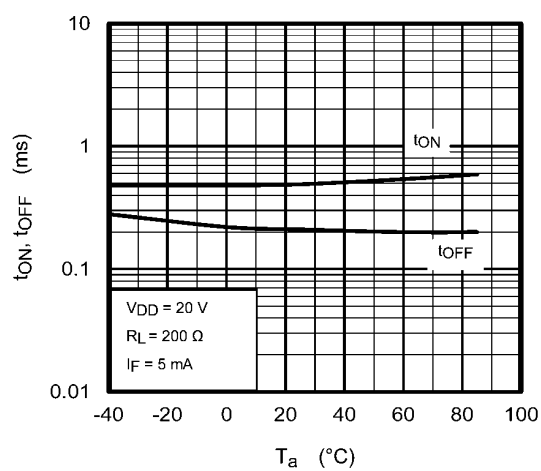
Fig. 14.1.8 t_{ON} , t_{OFF} - T_a
