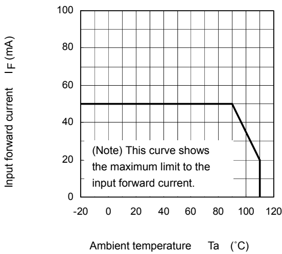
I_F - T_a
