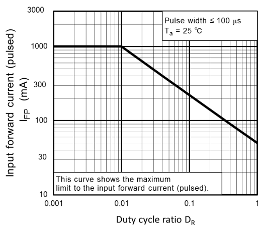
Fig. 12.4 I_{FP} - D_R
