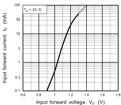
Fig. 12.3 I_F - V_F
