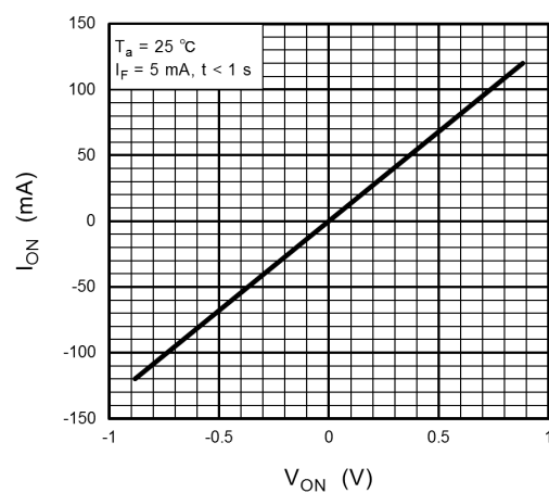
Fig. 12.4 I_{ON} - V_{ON}
