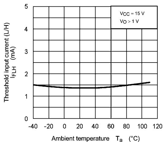
Fig. 12.2.4 I_{FLH} - T_a
