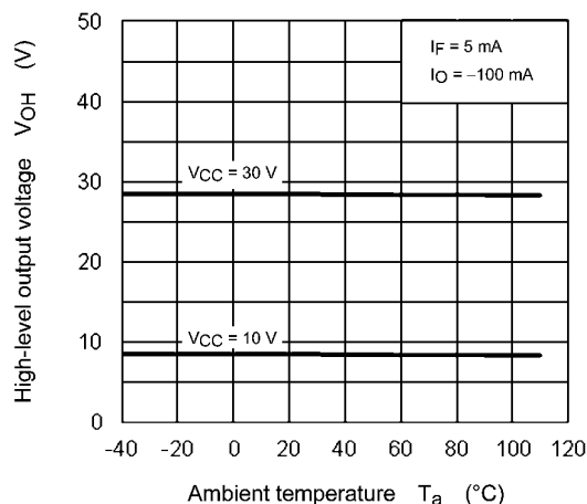
Fig. 12.2.8 V_{OH} - T_a
