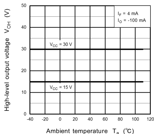
Fig. 12.2.8 V_{OH} - T_a
