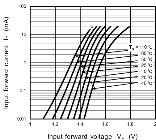
Fig. 12.2.1 I_F - V_F
