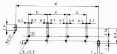
TM2RE-2408( 50 )
