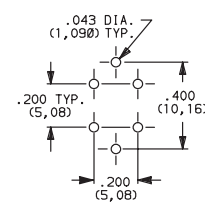
TP21SH9V3BE DPST
