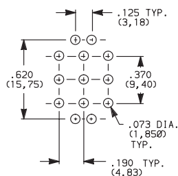
7301J1_BE2 3PDT
