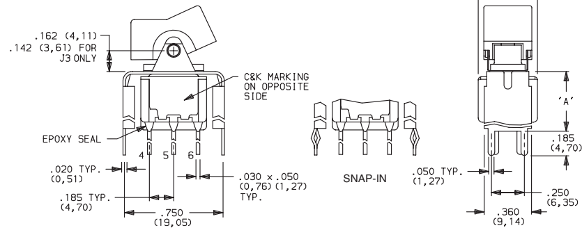
7201J1_BE2 DPDT
