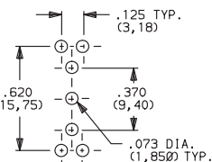
7101J1_BE2 SPDT
