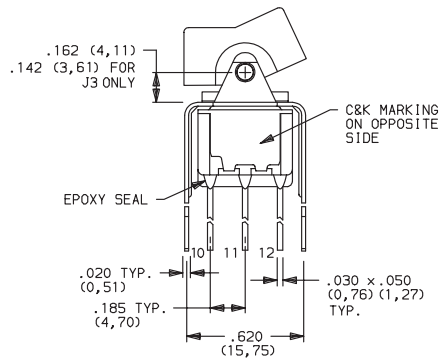
7401J1_BE2 4PDT
