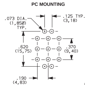
7301MD9_BE 3PDT
