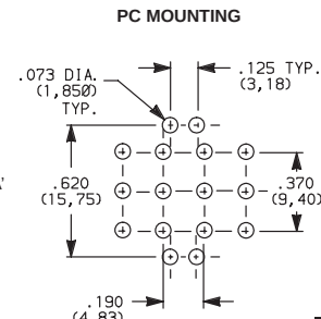
7401MD9_BE 4PDT
