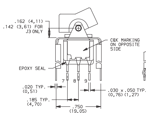
7301J1_BE2 3PDT
