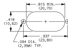
J8 Actuator
