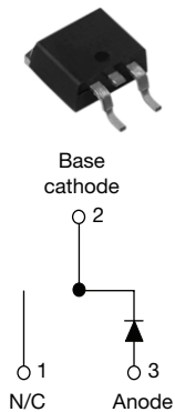
D²PAK
