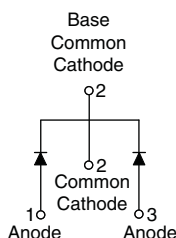
VS-30CTH02SPbF
