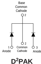
D 2 PAK
