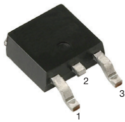
TO-252AA (D-PAK)
