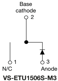
TO-263AB (D²PAK)
