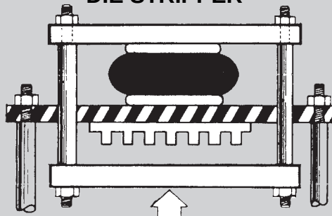
DIE STRIPPER
