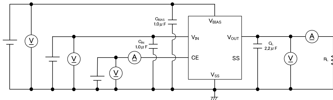
CIRCUIT④
