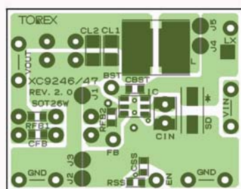
1 st Layer
