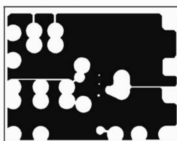
2 nd Layer
