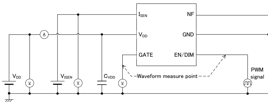
3) CIRCUIT③
