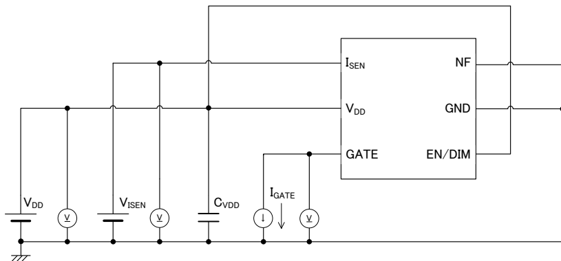
3) CIRCUIT③
