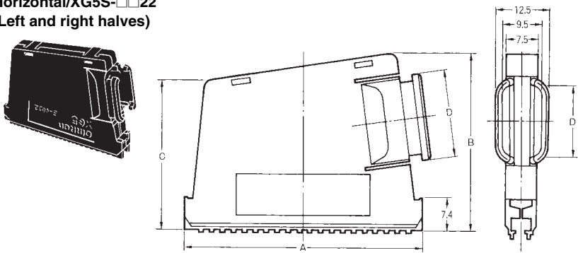
Dimensions
