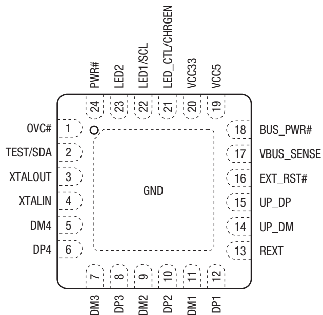
24-Pin QFN
