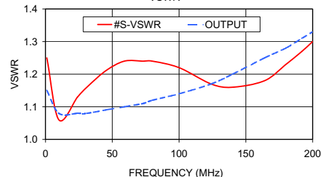
ZFSC-24-11-75 VSWR
