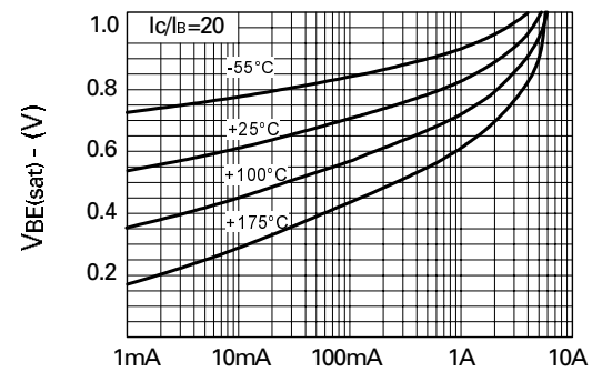
V_{BE(sat)} v I_C
