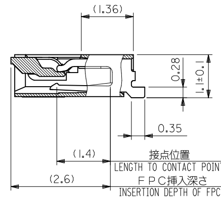
断面 W-W SECT. W-W 偶数極 (EVEN CKT)
