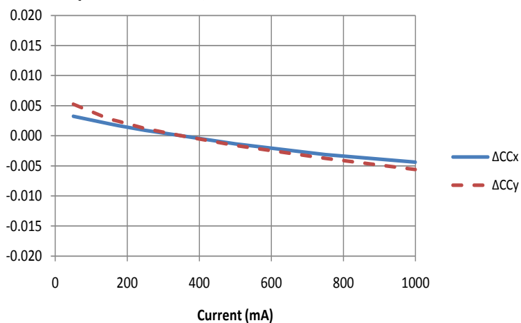
XLamp XM-L EZW LED, 12-V
