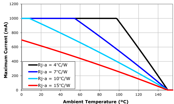
XLamp XM-L EZW LED, 12-V
