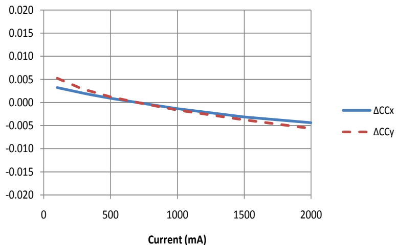
XLamp XM-L EZW LED, 6-V
