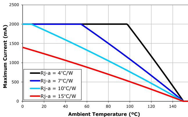
XLamp XM-L EZW LED, 6-V
