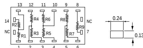
RMK 914N
