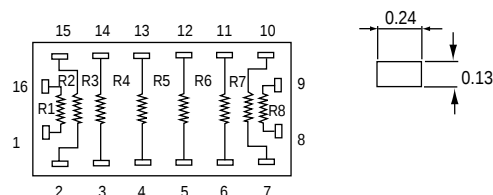
RMK 816N
