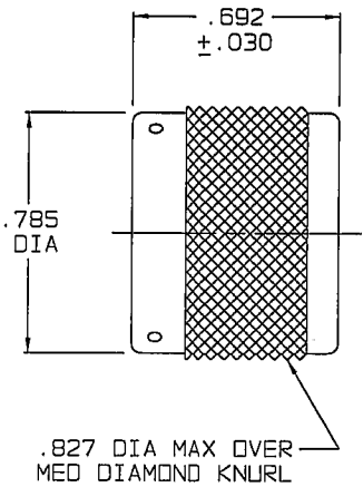
-1 SHOWN NO CHAIN/ROPE OR MOUNTING LUG
