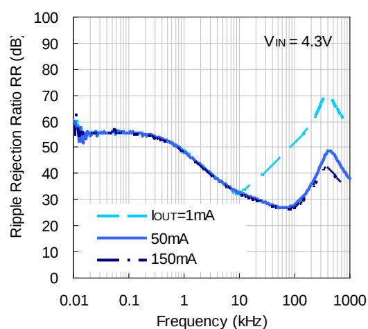
R1513S331B/D
