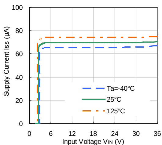
R1513S501B/D
