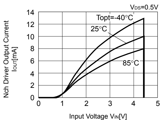
R3130N44xx
