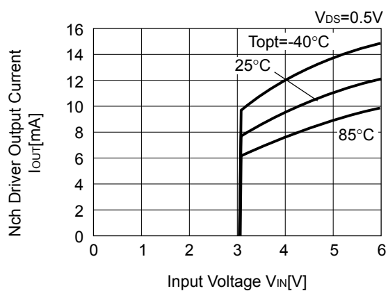
R3131N30xx8
