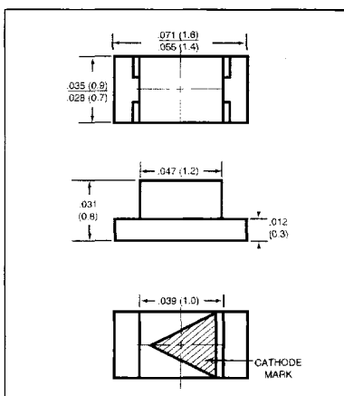
0603 Package
