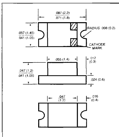
0805 Package
