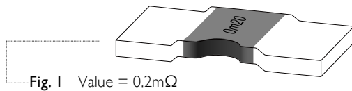
Fig. 1 Value = 0.2mΩ
