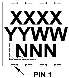
8-Lead UDFN (3x3x0.9 mm)
