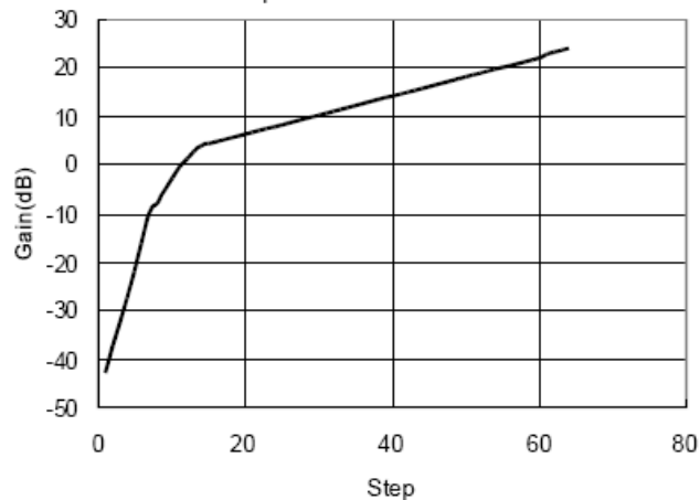
18. Gain Step
