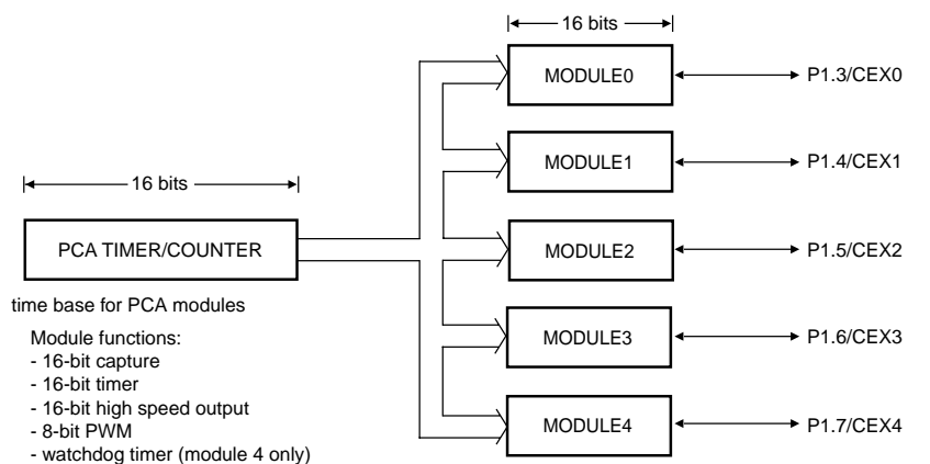
Fig 20. Programmable counter array
