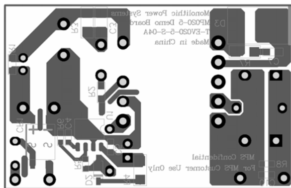
Bottom Layer
