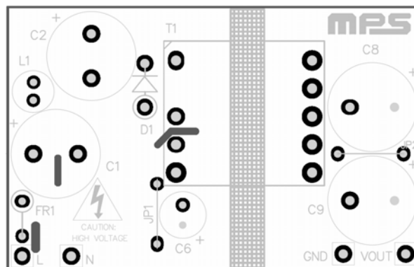
Top Layer
