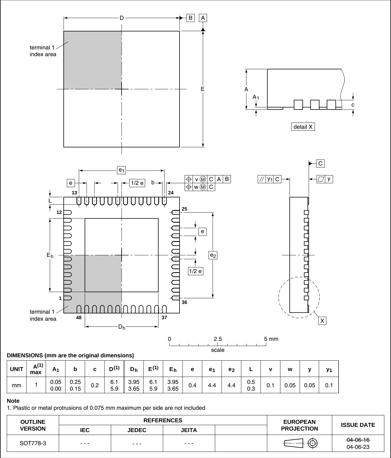
Fig 22. Package outline SOT778-3 (HVQFN48)
